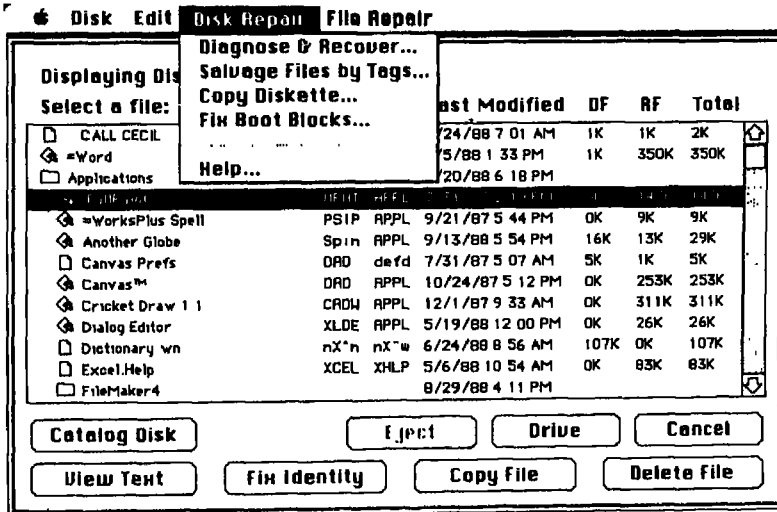
شكل (٢-١٢) : 1st Aid Kit ، هو وسيلة أخرى قادرة على استعادة الملفات والأقراص .
